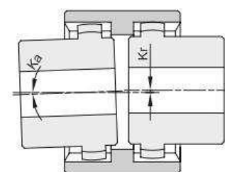
Угловое/Радиальное смещение
