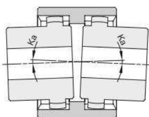
Угловое смещение
