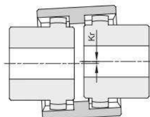
Радиальное смещение
